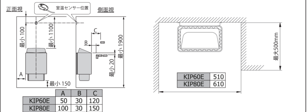
【サウナヒーターの離隔距離 [mm] と室温センサー位置】 【奥まった場所に取り付ける際のサウナヒーターの離隔距離 [mm]】
